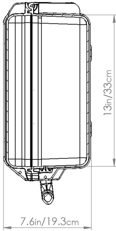
SECTION B-B SCALE 1 : 5
