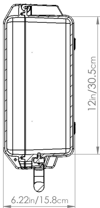
SECTION A-A SCALE 1 : 5
