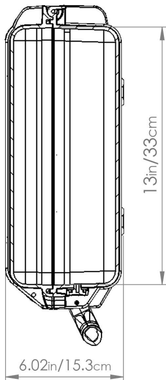
SECTION B-B SCALE 1 : 5
