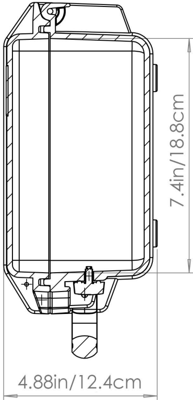
SECTION A-A SCALE 1 : 3
