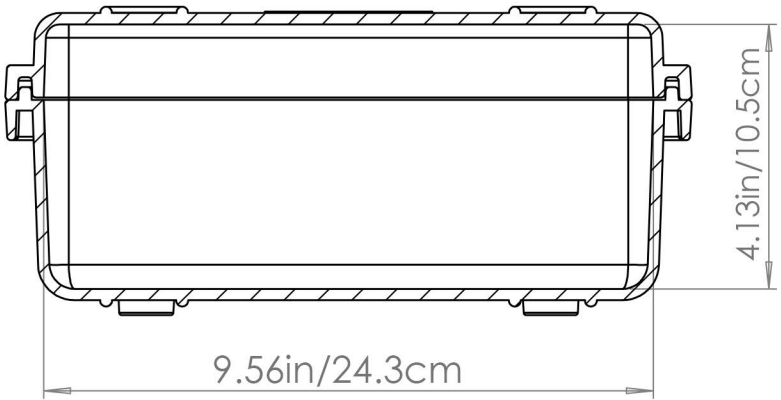
SECTION B-B SCALE 1 : 3
