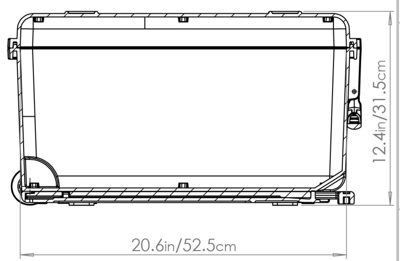
SECTION A-A SCALE 1 : 6
