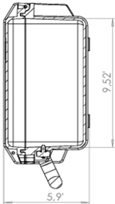
SECTION A-A SCALE 1 : 4
